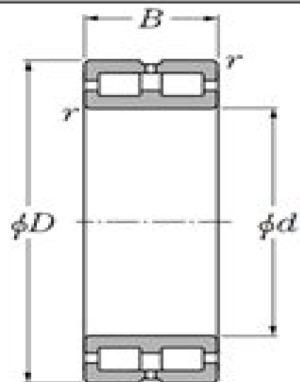
SL01 Type
