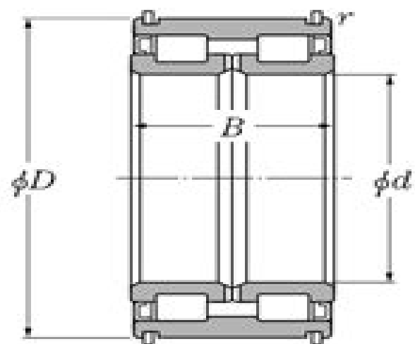
SL04 Type
