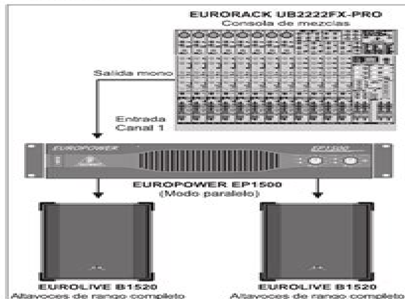
Fig. 3.3: Funcionamiento paralelo
