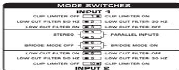
Fig. 3.2: Posiciones del interruptor DIP para el funcionamiento en dos canales
