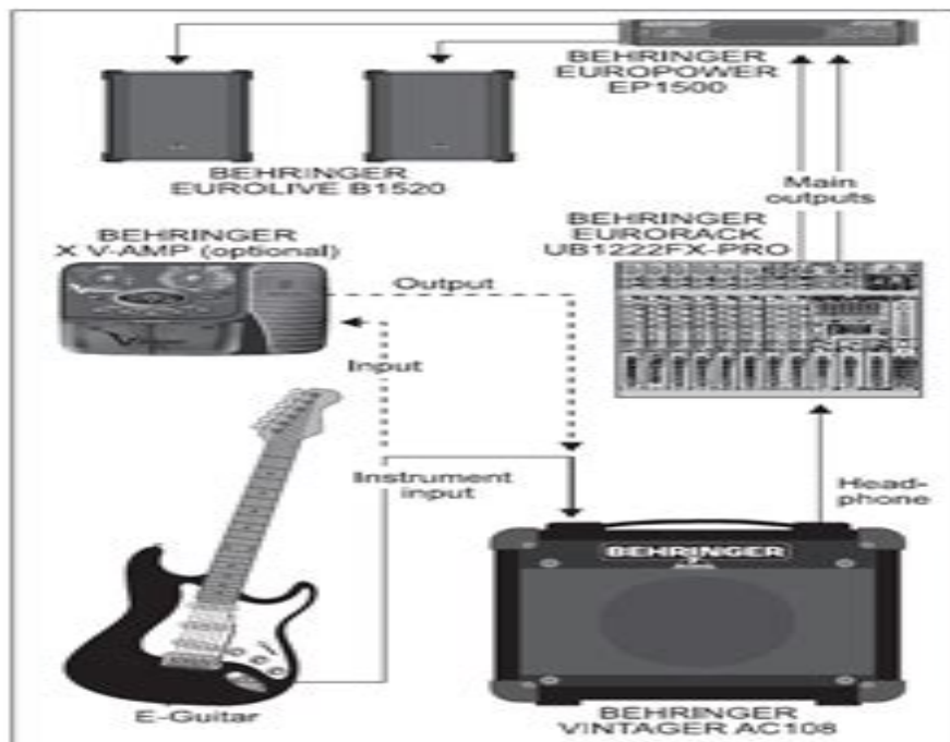
Fig. 2.2: Live setup
