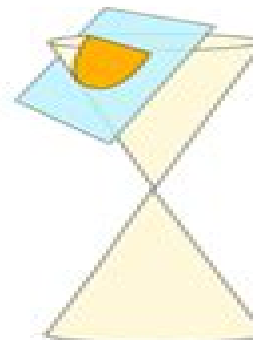
Parabola
