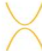
Hyperbola
