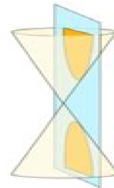
Hyperbola
