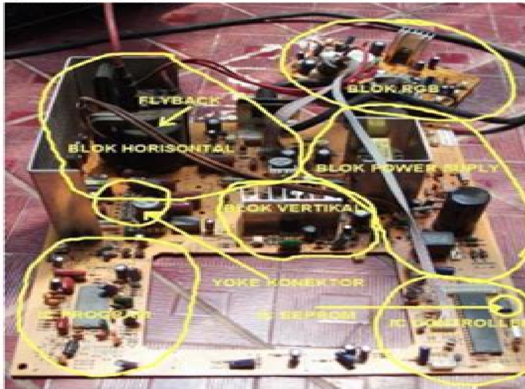
Gambar Bagian Blok TV
