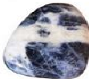
sodalite
