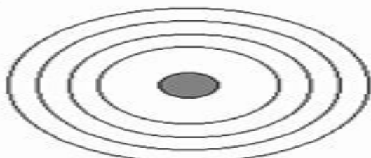
Sodium
