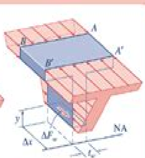
(d) A free-body diagram for determining web shear flow.
