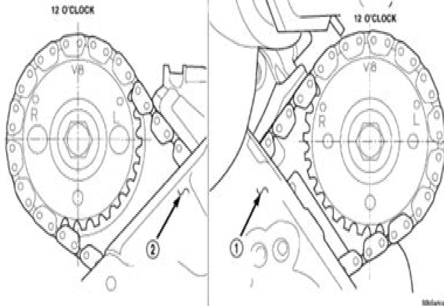
Fig. 121 Camshaft Sprocket V8 Marks
