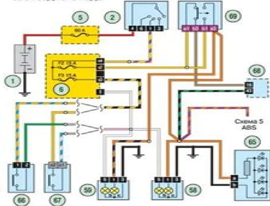
Корректоры фар
