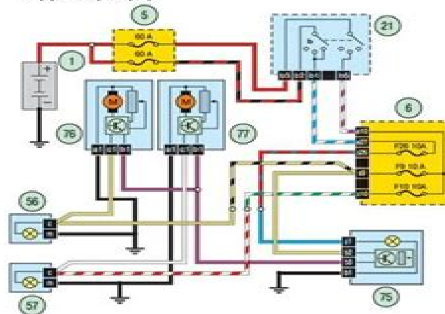
Корректоры фар
