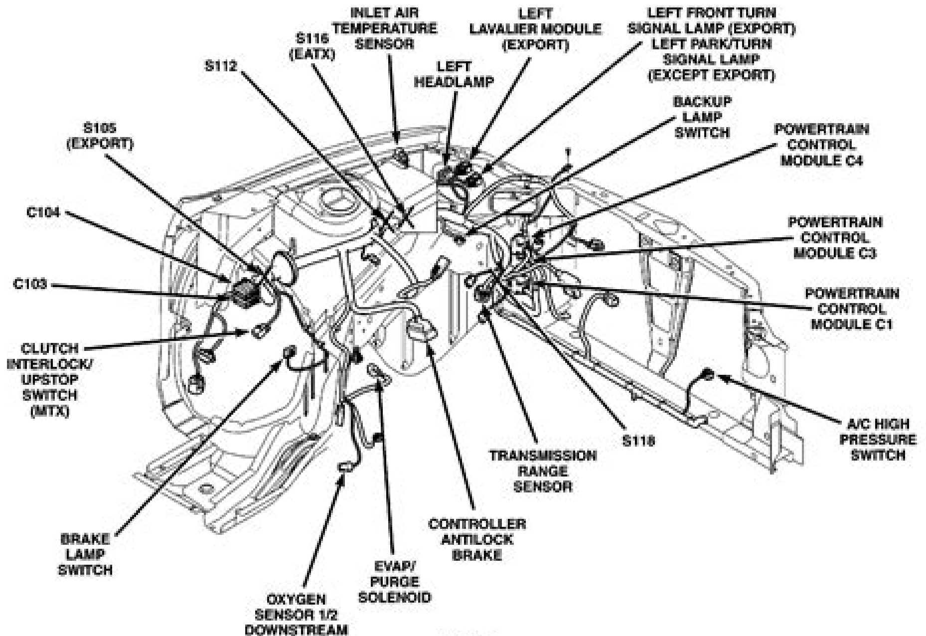
VIEW Y
