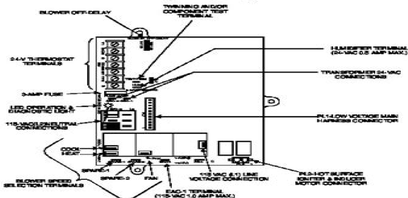
Fig. 11—Field Wiring
