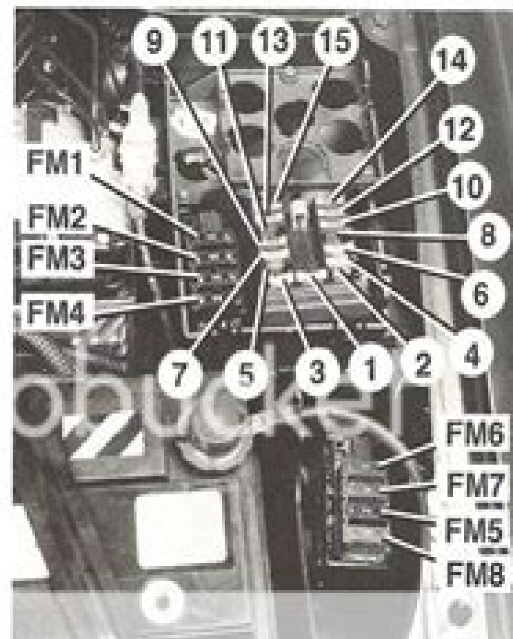
Implantation des fusibles dans le compartiment moteur.
