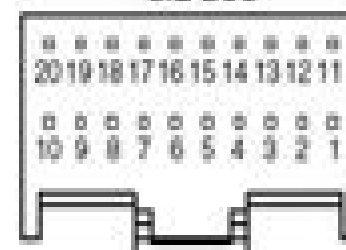
SIE-BUS
