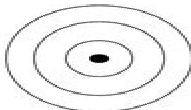
Silicon (Si) _____
