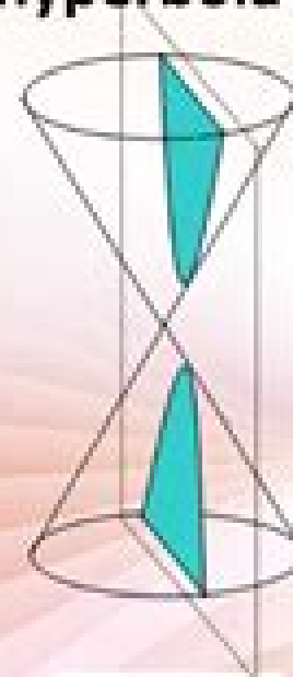
HYPERBOLA
