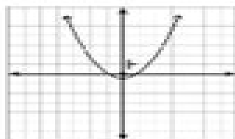
Parabola
