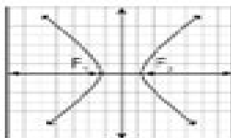
Hyperbola
