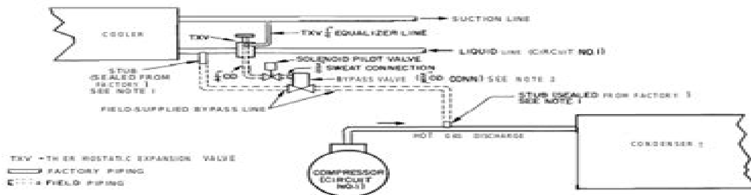
Fig. 1 — Schematic Piping: 30HK,HL015-060; 30GT015-035
