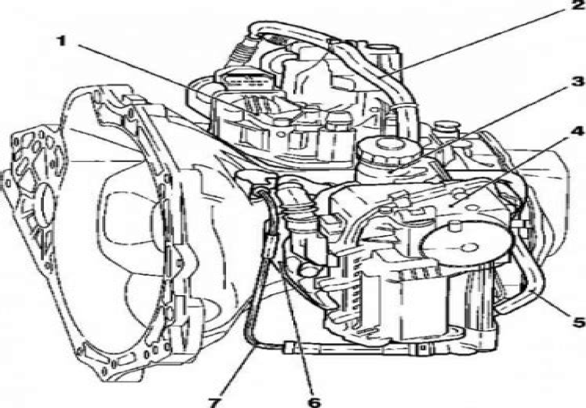
Коробка передач Easytronic: 1 – модуль переключения передач; 2 – кабельный канал; 3 – бак с тормозной жидкостью; 4 – блок управления сцеплением; 5 – шланг гидравлического контура сцепления; 6 – кронштейн крепления блока управления сцеплением; 7 – возвратный гидравлический контур
