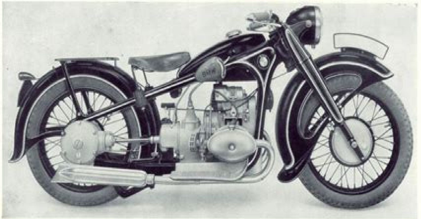
R 17-Maschine von der Antriebsseite aus
