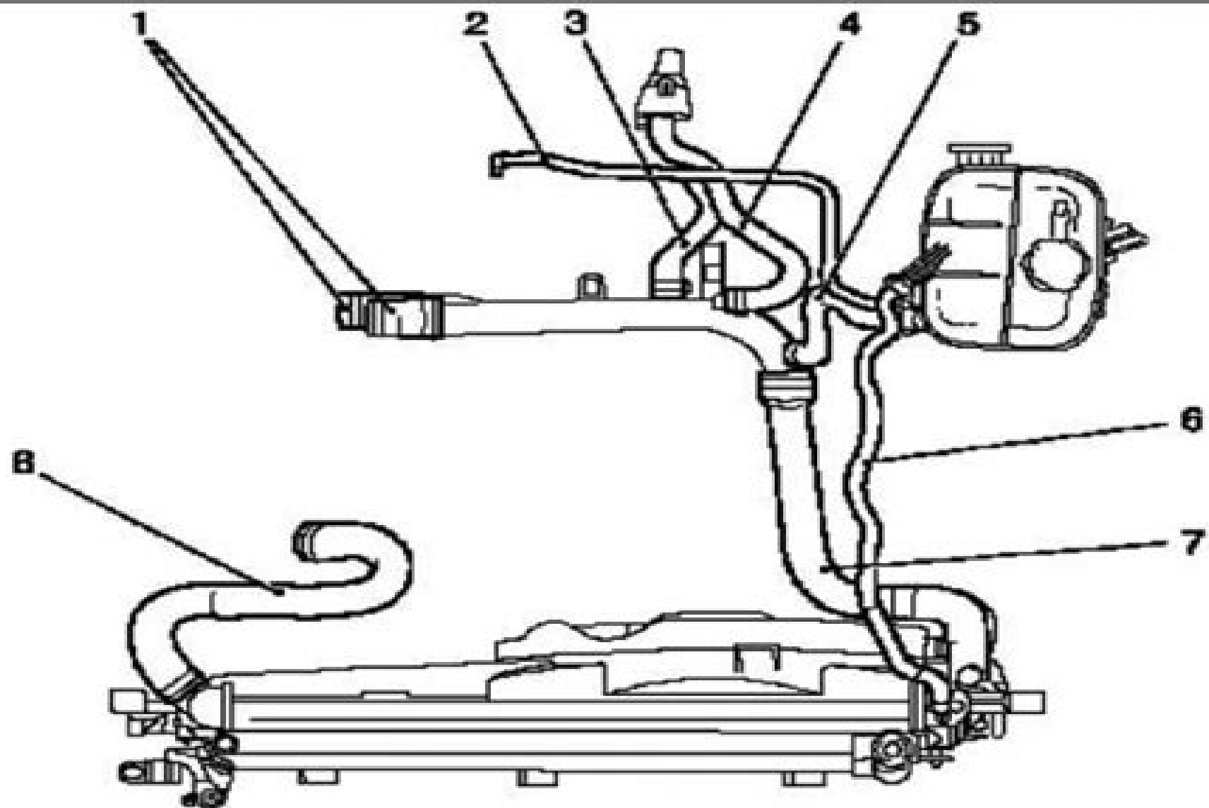
Компоненты системы охлаждения (двигатели 1,4–1,6 л): 1 – расширительный бачок охлаждающей жидкости; 2 – соединительный шланг, от расширительного бачка к радиатору; 3 – радиатор; 4 – коленчатый патрубок нижнего шланга радиатора; 5 – соединительный патрубок к холодильнику рециркуляции отработавших газов; 6 – трубка охлаждения рециркуляции отработанных газов; 7 – терморегулятор; 8 – возвратный шланг, радиатор отопителя; 9 – подающий шланг, радиатор отопителя; 10 – соединительный шланг, от штуцера к расширительному бачку; 11 – соединительный шланг, от контура охлаждения двигателя к расширительному бачку
