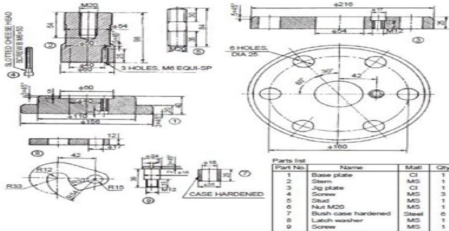
Fig. 18.24 Drill Rig
