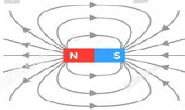
Bar magnet
