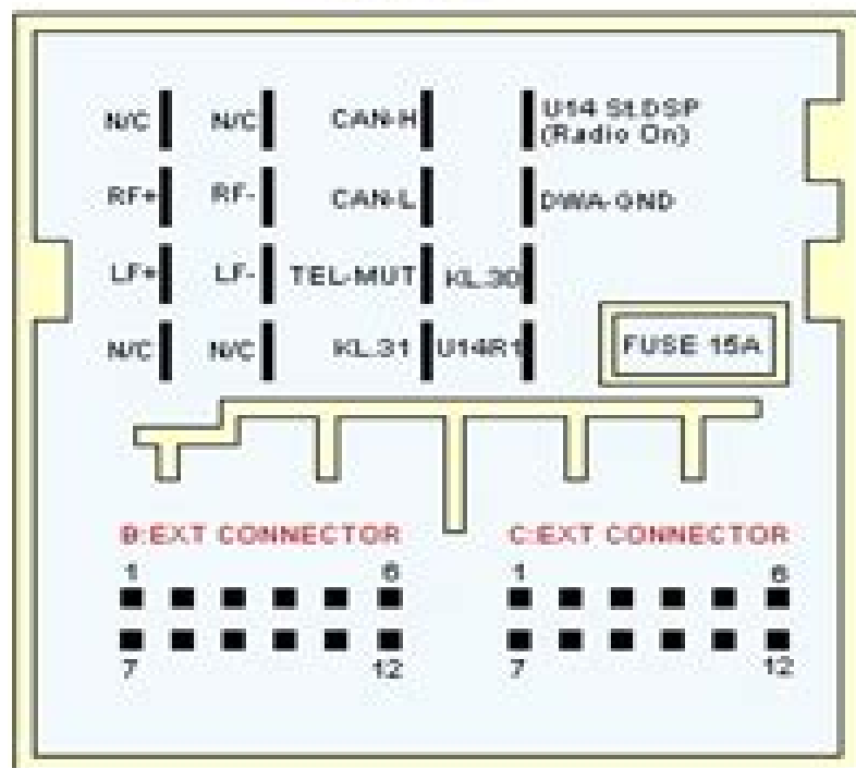
Распиновка разъёмов "B" "C"
