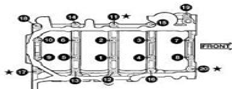
Fig. 55 Bedplate Bolts
