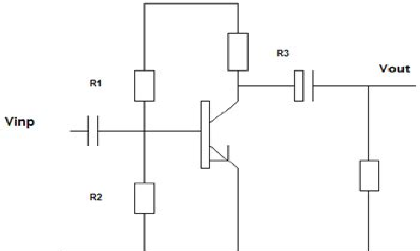
BJT Amplifier
