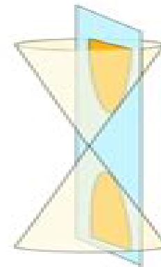
Hyperbola
