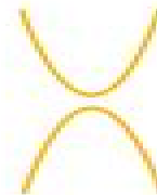
Hyperbola
