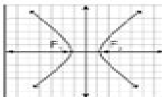
Hyperbola
