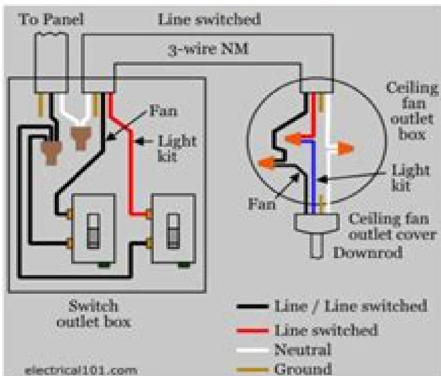
Ceiling Fan Switch Wiring Diagram 2
