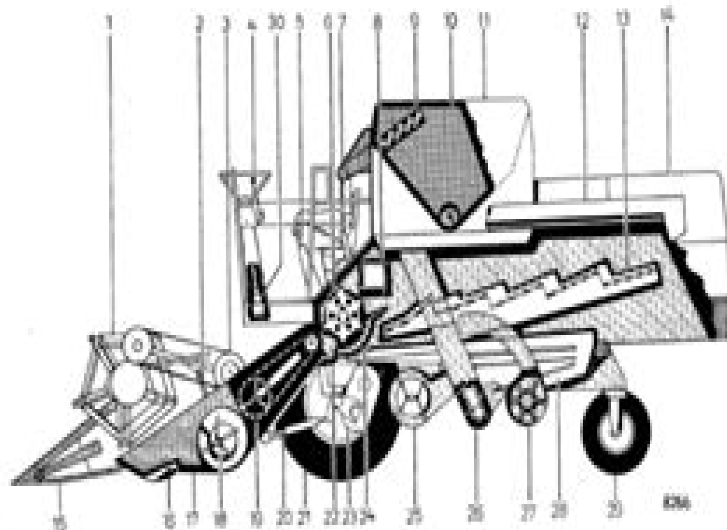
Schnittbild M 600
