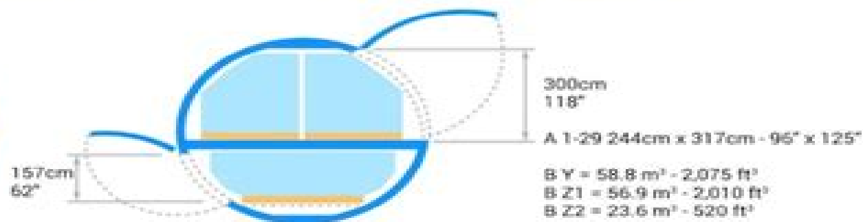
Boeing B747-200F
