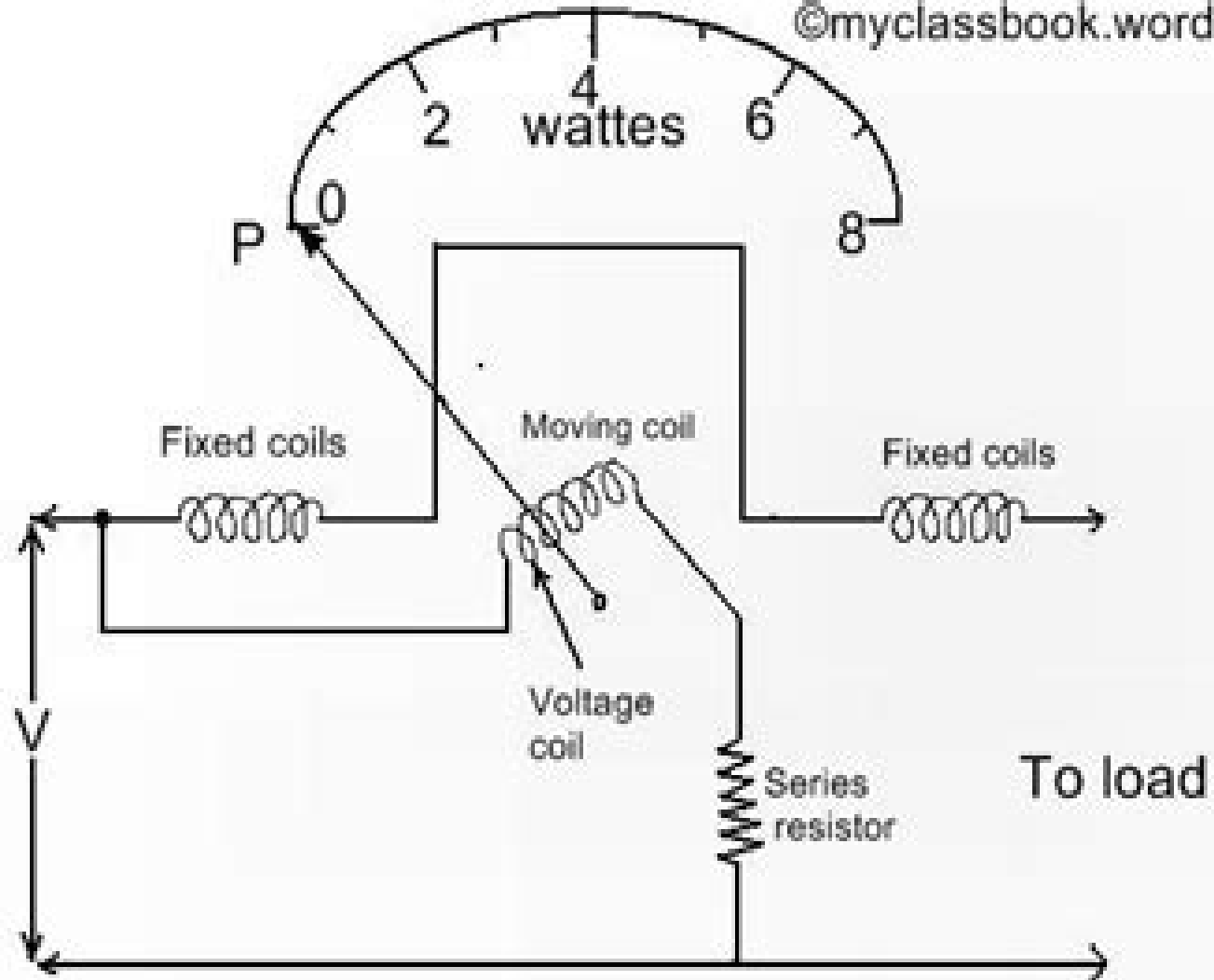
Dynamometer type Wattmeter
