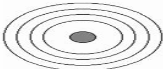
Alumunium
