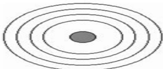
Calcium
