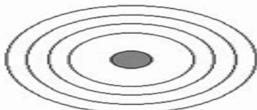
Helium
