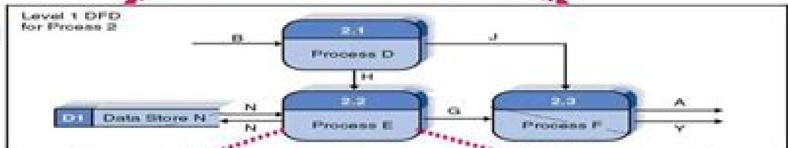
Level 1 DFD
