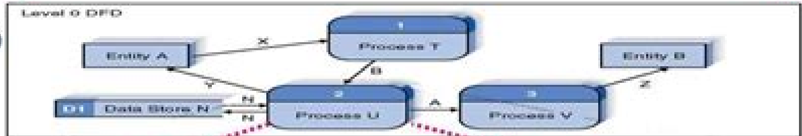
Level 0 DFD
