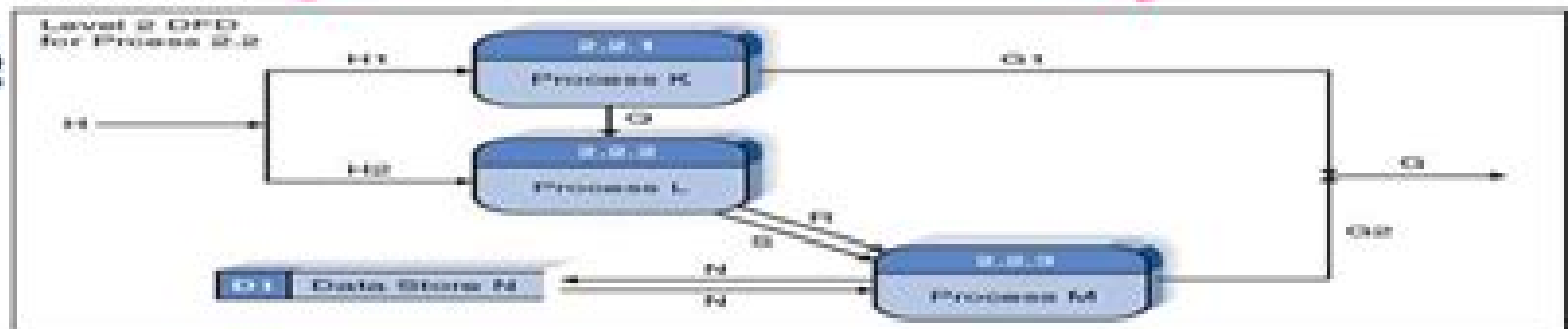
Level 2 DFD
