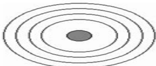
Calcium
