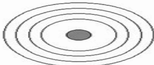
Helium
