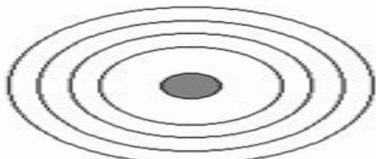
Alumunium
