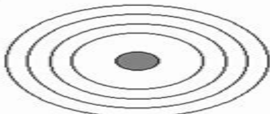
Sodium
