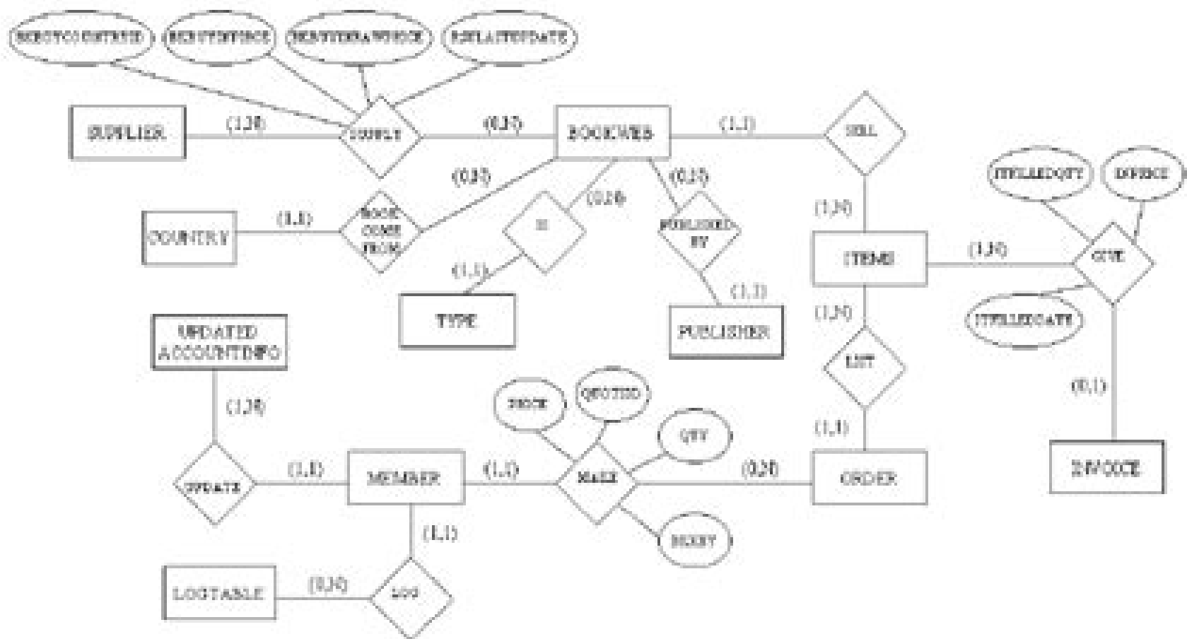
ER Diagram
