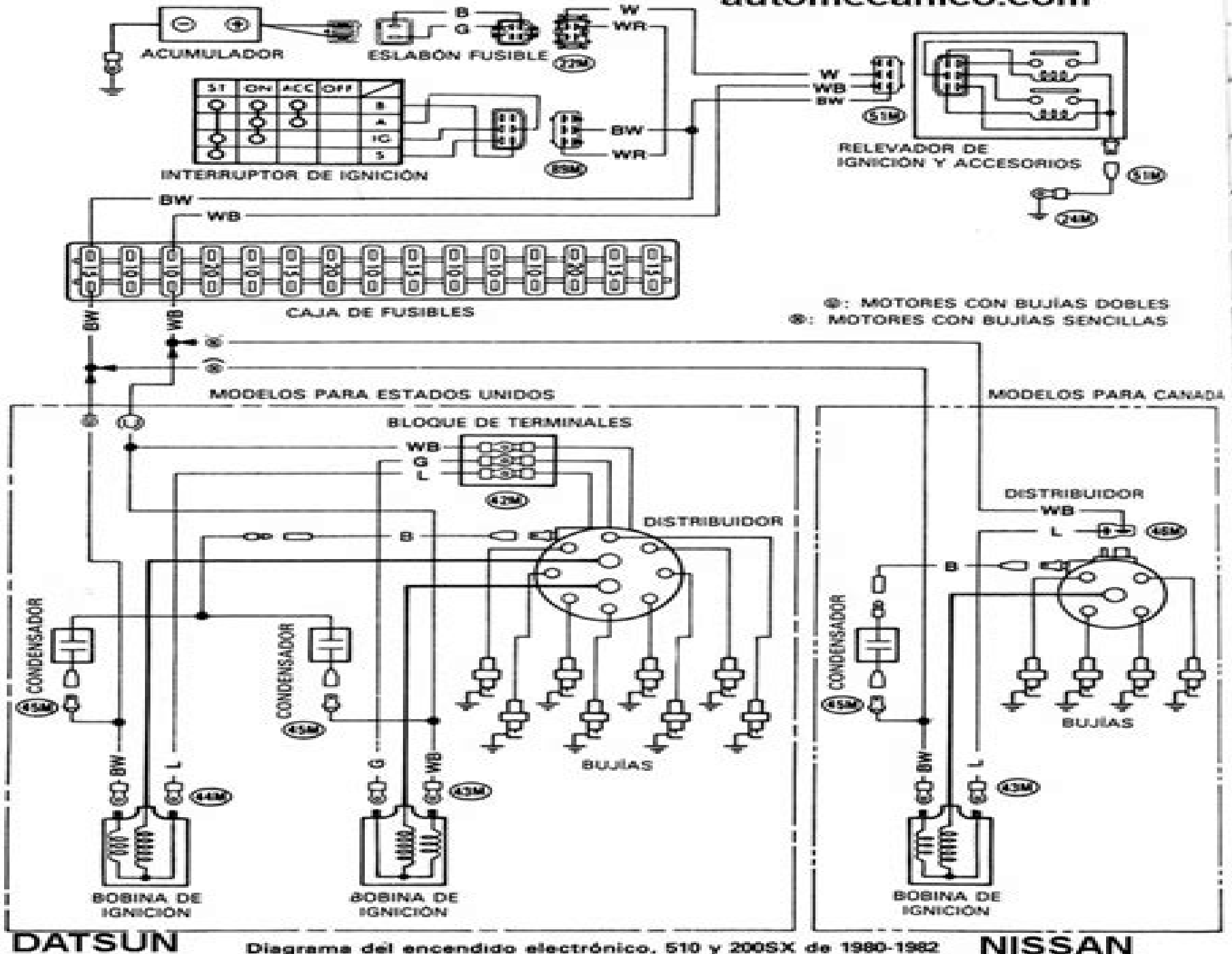
Diagrama del encendido electrónico, 510 y 200SX de 1980-1982
