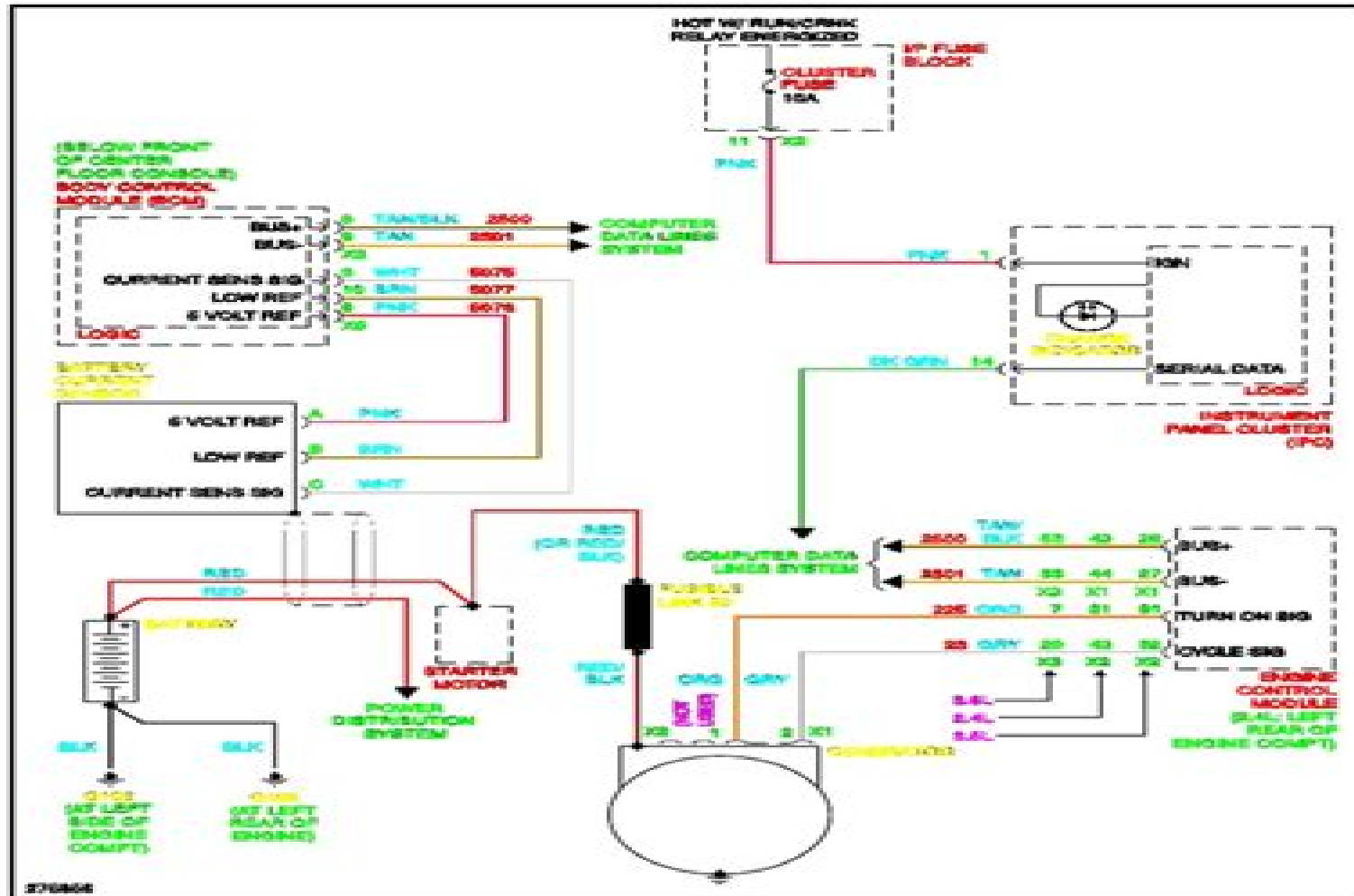
2.4L VIN P, Charging Wiring Diagram
