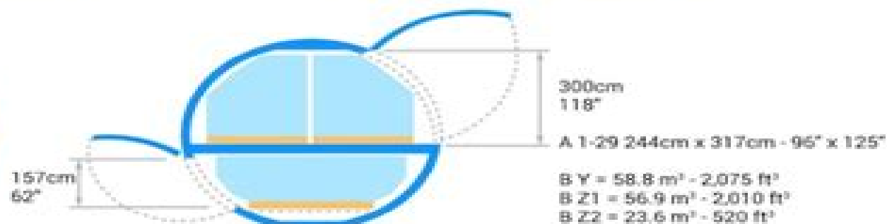
Boeing B747-200F
