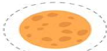
Venus
