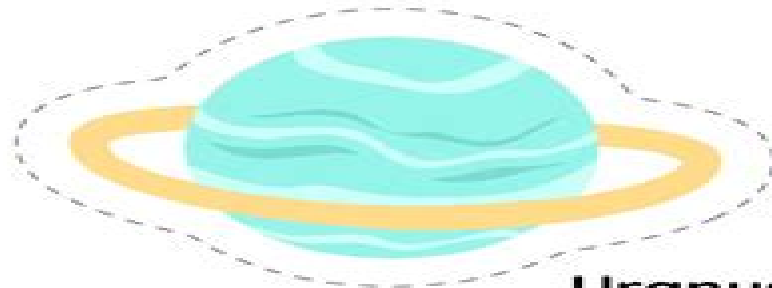
Uranus
