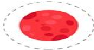
Mars
