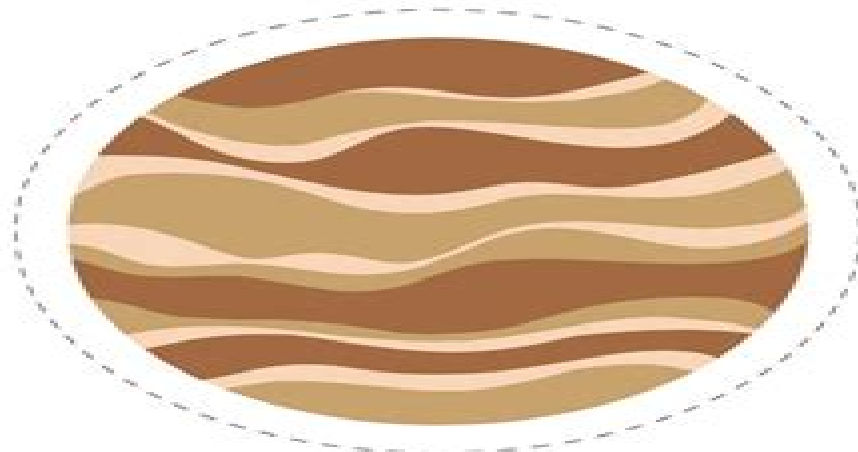
Jupiter
